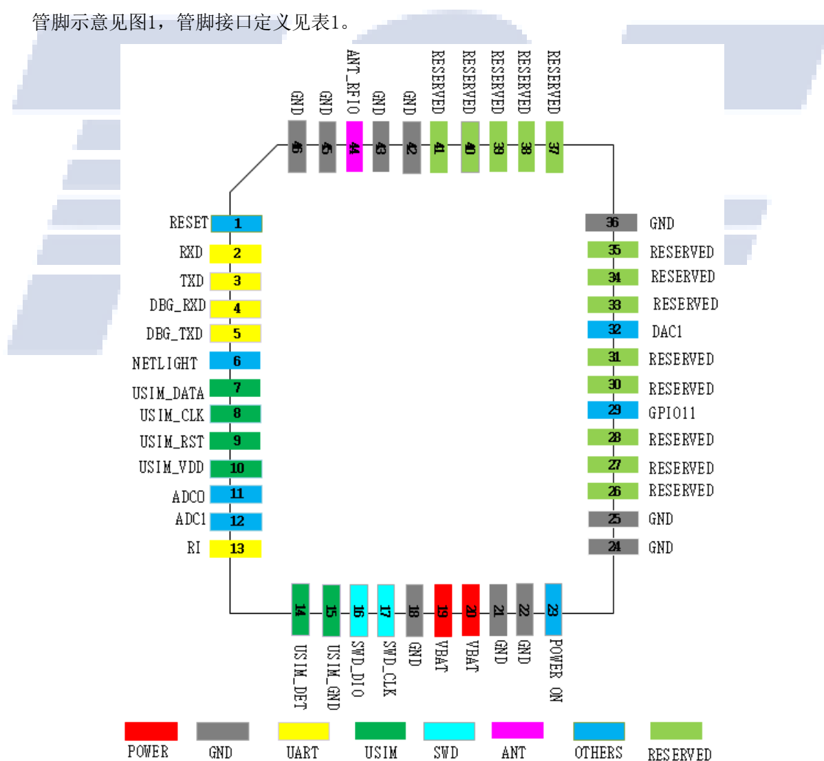
图1 管脚示意图
